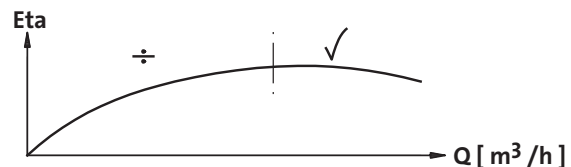
Рис. 23 Максимальный КПД
