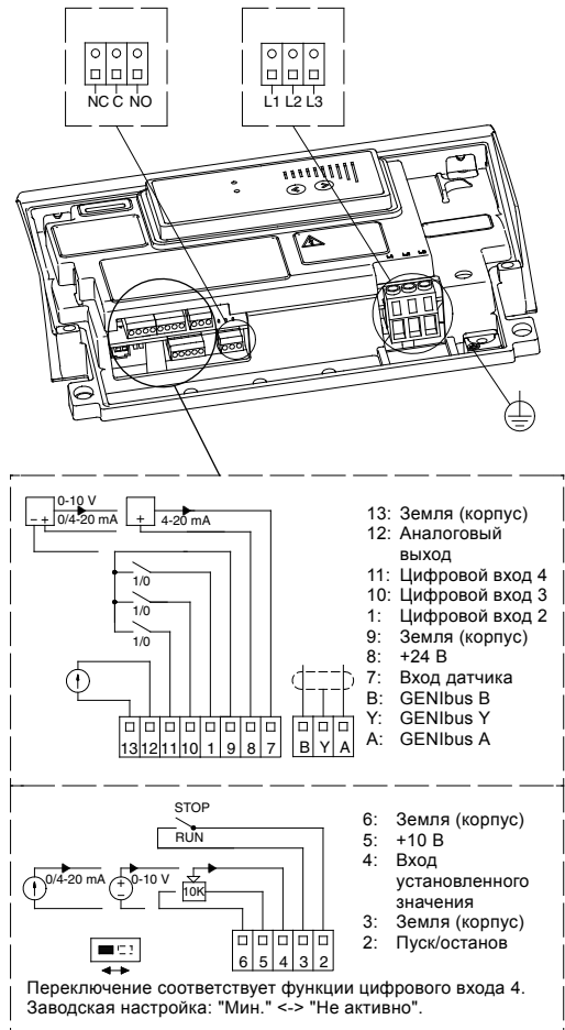
Рис. 6 Клеммы соединений, расширенный модуль входа/выхода
