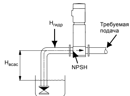
Рис. 24 Размерные данные
