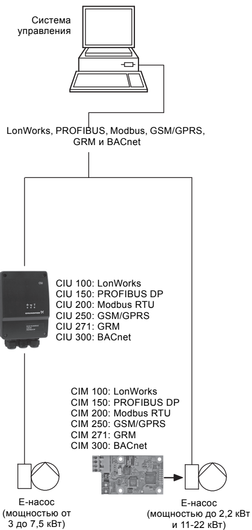
Рис. 14 Структура центральной системы управления
